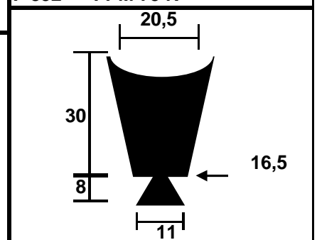
F 833 IIR 70 N
