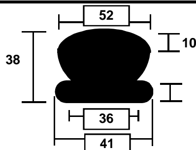
F1319 NR 75 N
