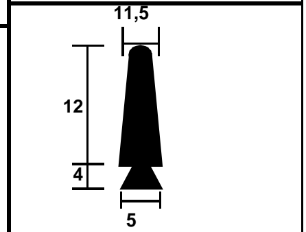
F 852 FPM 75 N
