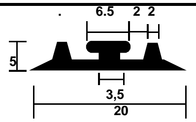
F 722 CR 65 N
